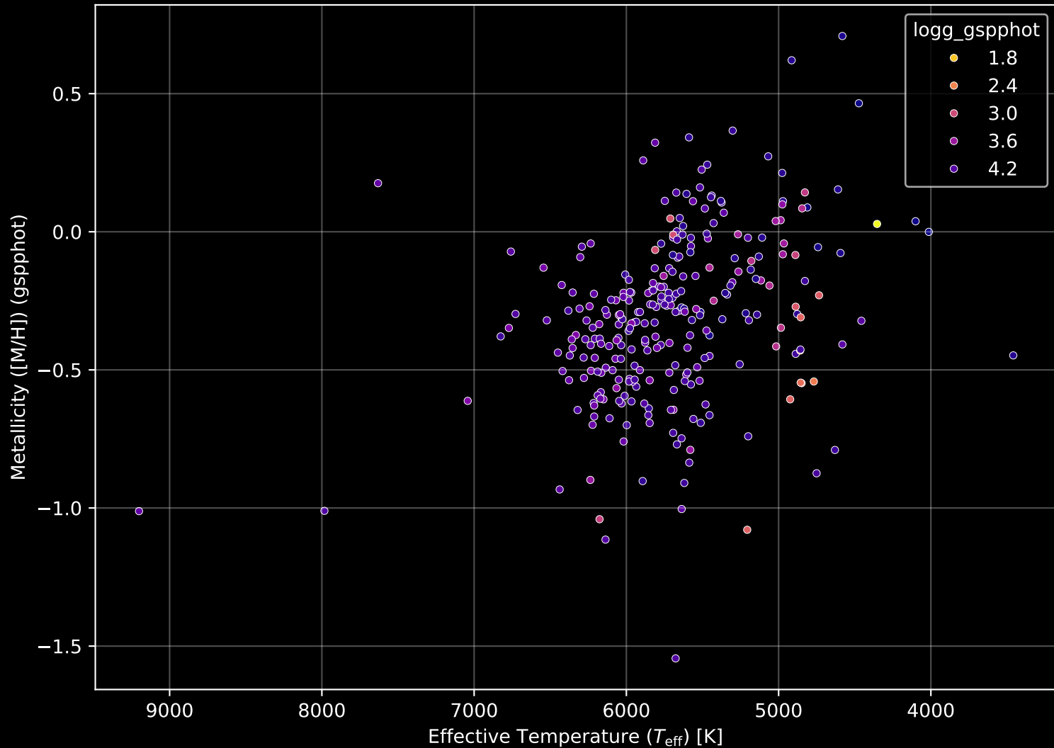
GALAH DR4 Field: [466] Stellar Population Parameters (n= 280)
