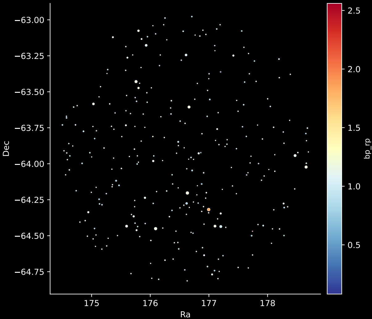
GALAH DR4 Field: [466] Stars: 280
