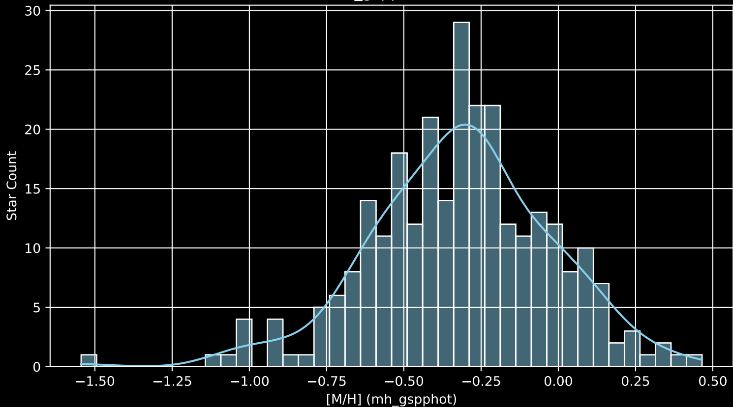
GALAH DR4 Field: [466] [M/H] (mh_gspphot) (n= 278)
