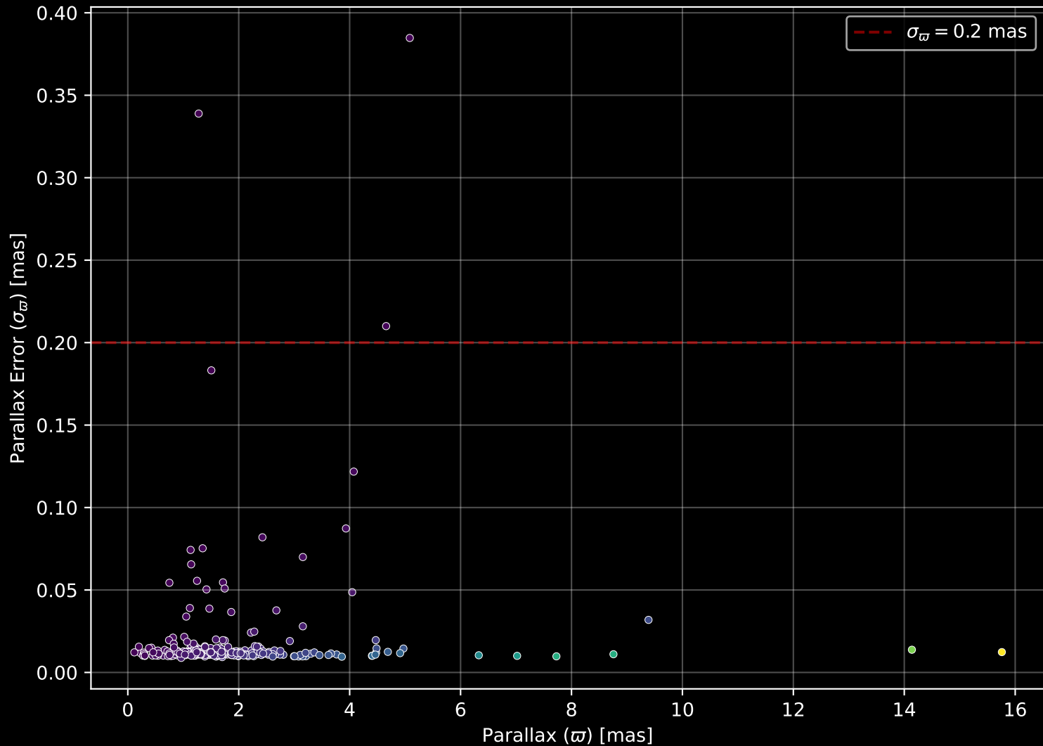
GALAH DR4 Field: [466] Parallax Quality (n= 280)
